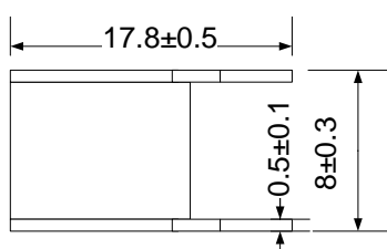
图 2: K2 电极片
